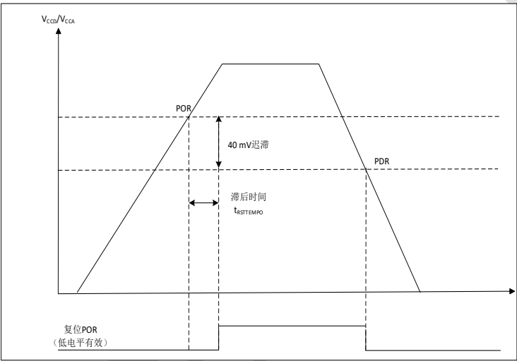
图 2-3 POR/PDR 阈值
