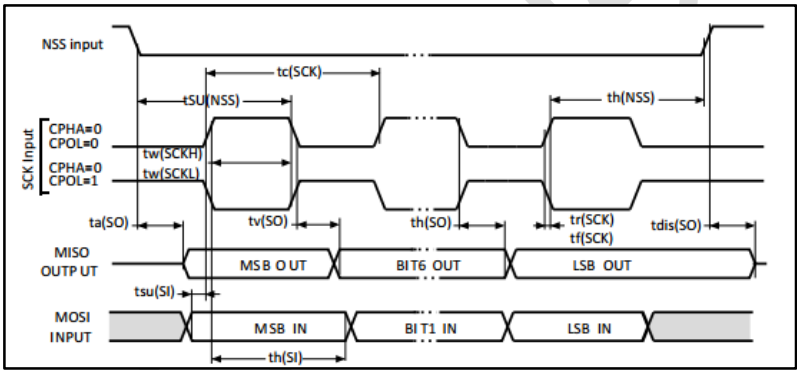
图 5-6 SPI 时序图-从模式且 CPHA = 0
