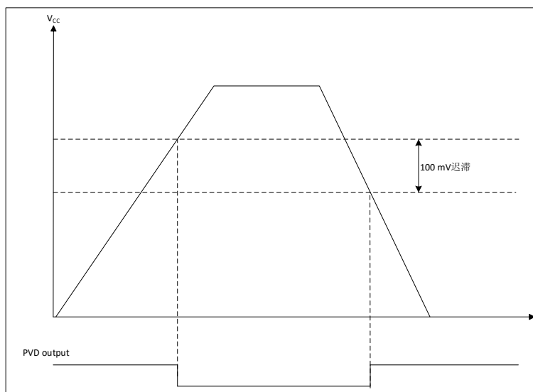
图 2-4 PVD 阈值
