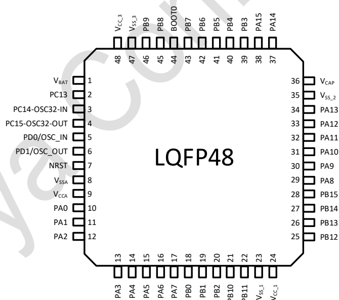
图 3-4 LQFP48 PY32F403C1XT Pinout1 (Top View)
