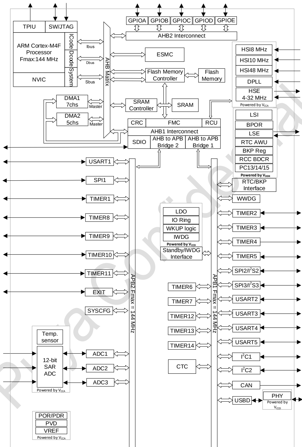
图 1-1 功能模块
