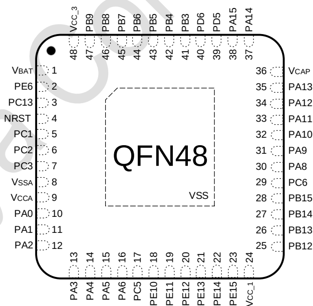
图 3-6 QFN48 PY32F403C1xU Pinout1 (Top View)
