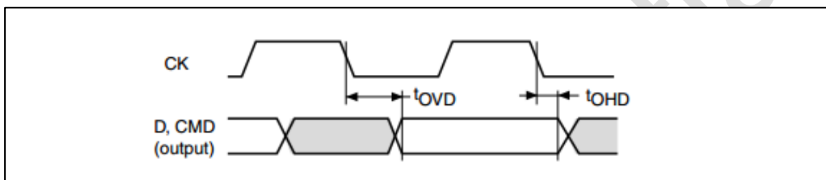
图 5-13 SD 默认模式
