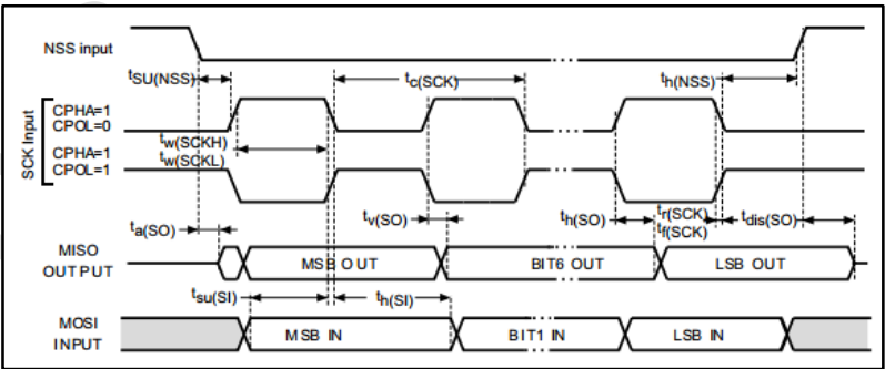
图 5-7 SPI 时序图-从模式且 CPHA = 1(1)
