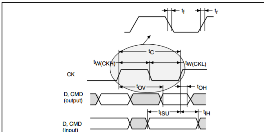
图 5-12 SDIO 高速模式
